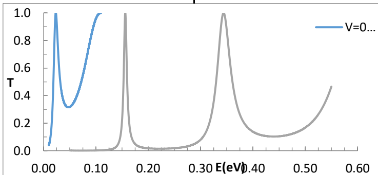
شكل (5) أثر تغيير ارتفاع الحاجز (V) على منحنيات النفاذية كدالة في الطاقة لحاجزين، w=10nm و b_w=2nm
