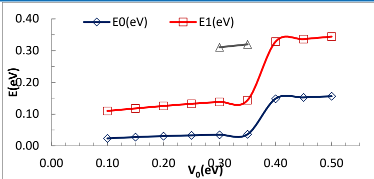
شكل (6): أثر تغيير ارتفاع حاجز الجهد على مستويات الطاقة لحاجزين b_w=2\text{nm} و w_w=10\text{nm}
