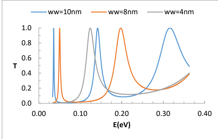
شكل (2) أثر تغير عرض البئر على منحنيات معامل النفاذية لحاجزين، b_w=2\text{nm} وارتفاع حاجز الجهد 0.33\text{eV}
