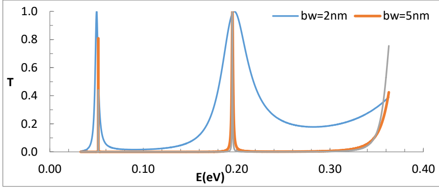
شكل (4): أثر تغيير سمك الحاجز على منحنيات النفاذية كدالة في الطاقة لحاجزين، w=8nm وارتفاع حاجز الجهد 0.33eV و x=0.1 .
