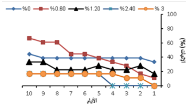
الشكل (1). تأثير ملوحة كلوريد الصوديوم على النسبة المئوية للإنبات في الذرة البيضاء خلال عشرة أيام من الإنبات.
