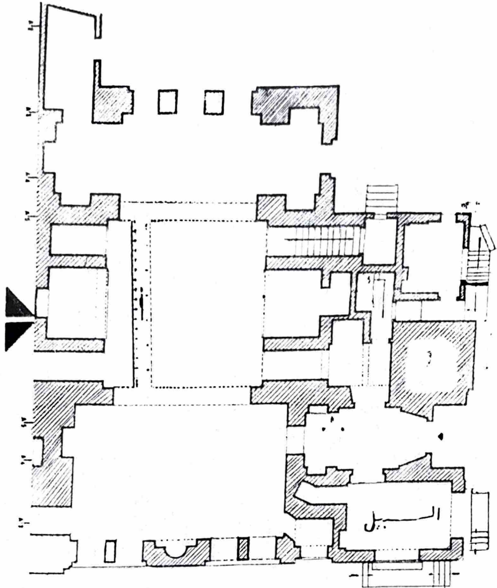
مخطط أفقي لمدرسة جميع السطاح قايماي ٨٧٧ : ٨٧٩ هـ - ١٤٧٩ : ١٤٧٩ م "بقرافة قايماي من القاهرة" صبيحة السيل الذي أوجده المعمار بالناحية الشرقية للمدرسة حتى يفتح به سلكي تسهيل . نقلا من : أرشف قسم الرسم بمصلحة الآثار بالقاهرة .
