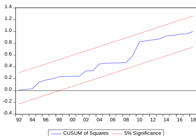
الشكل البياني (2): المجموع التراكمي لمربعات البواقي
