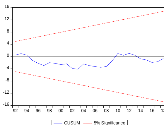
الشكل البياني (1): المجموع التراكمي للبواقي
