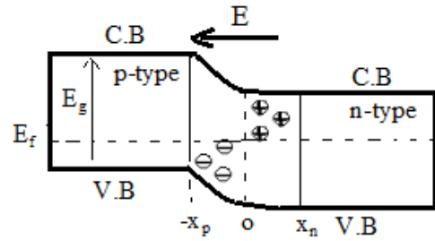
ب- مستويات الطاقة و المجال الكهربائي الناشئ
