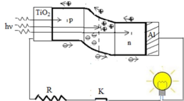
شكل 2: تحويل الإشعاع الشمسي إلى تيار كهربى بالوصلة p-n
