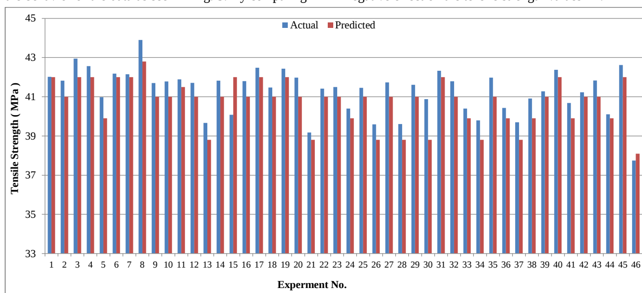
Fig. 5. Actual Vs. Predicted Values for Plan II.
