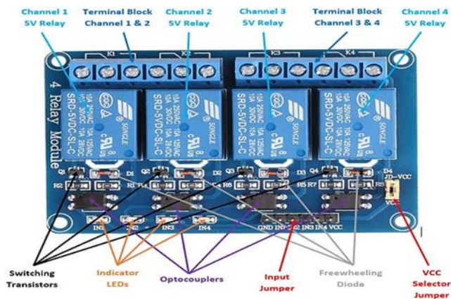
Fig. 5. Relay module 4x4.
